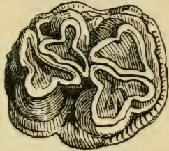
Fig. 435.
